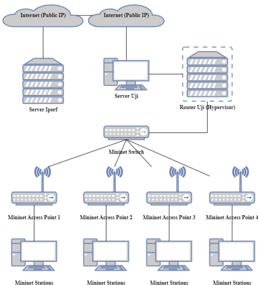
Gambar 1. Topologi Jaringan Simulasi
