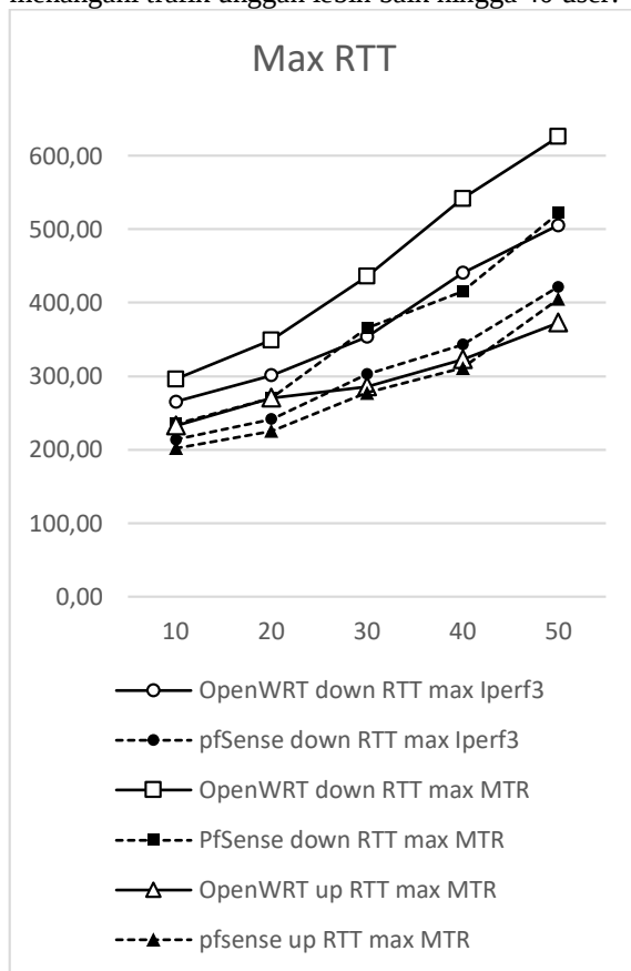
Gambar 7. RTT Maksimum RTT pada OpenWRT dan PfSense.
