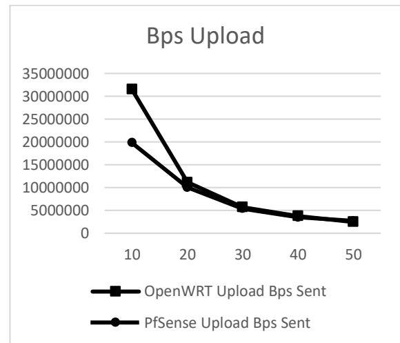
Gambar 4. Grafik Throughput Unggah.
