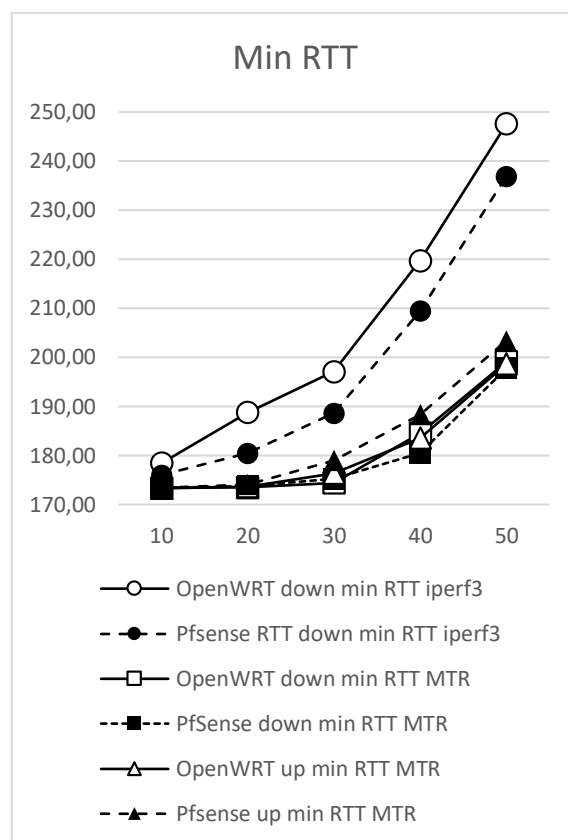
Gambar 6. RTT Minimum RTT pada OpenWRT dan PfSense
